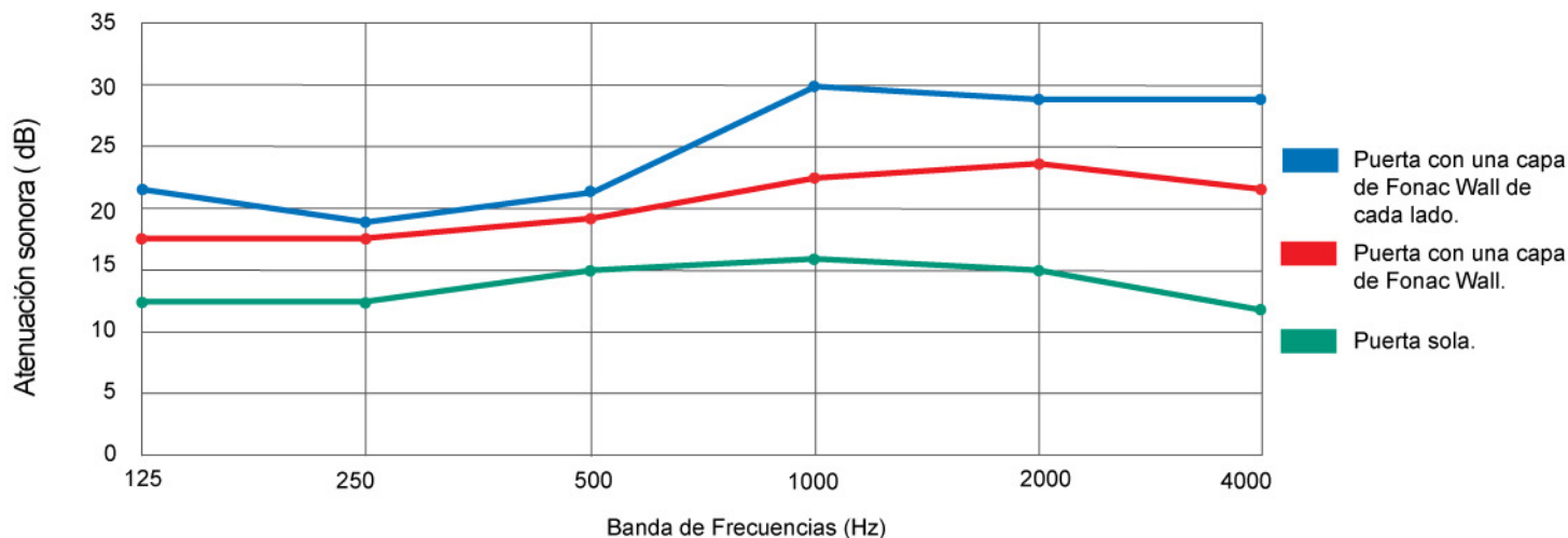
Curvas de atenuación sonora
